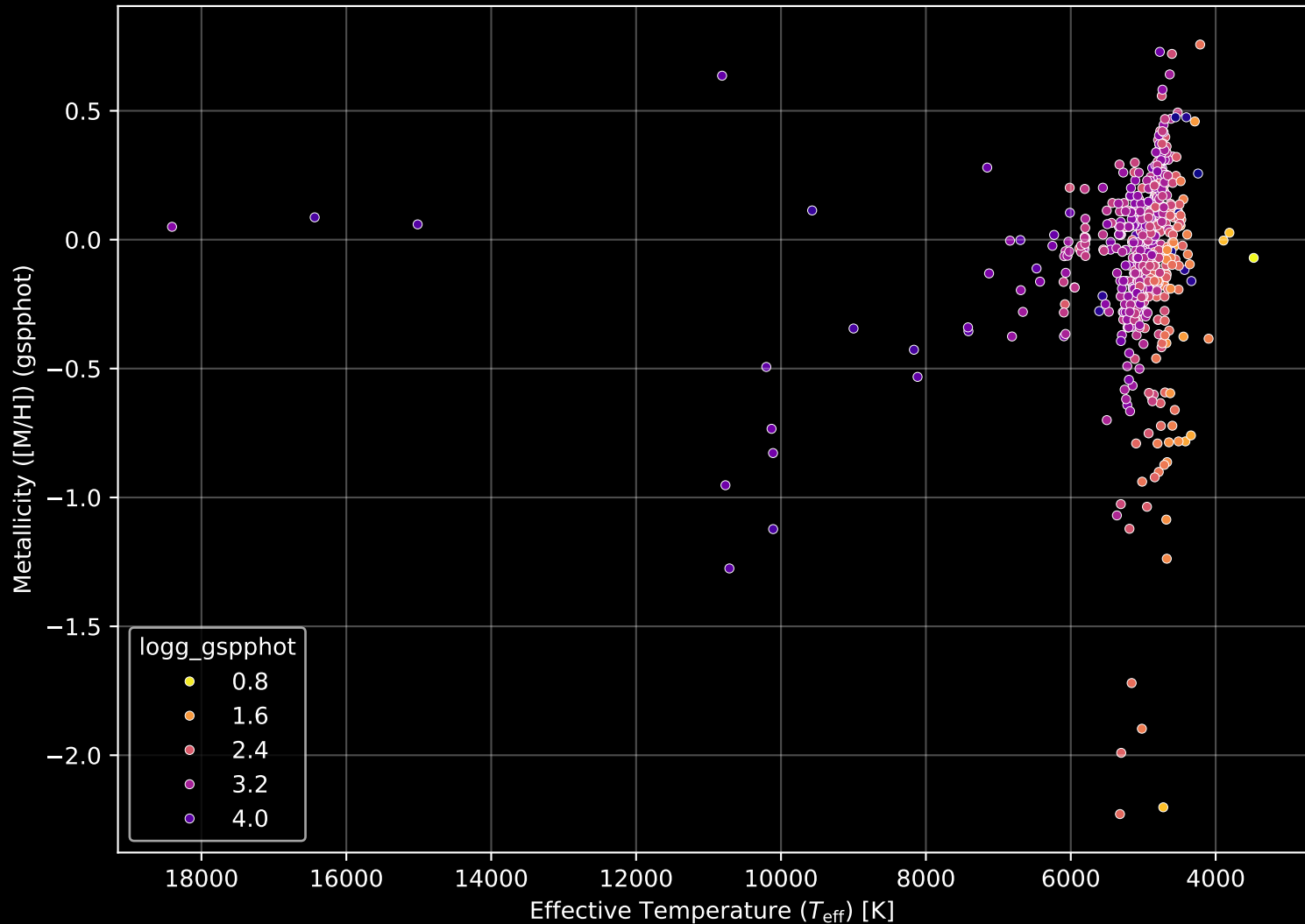
APOGEE DR17 Field: [094+06] Stellar Population Parameters (n= 571)
